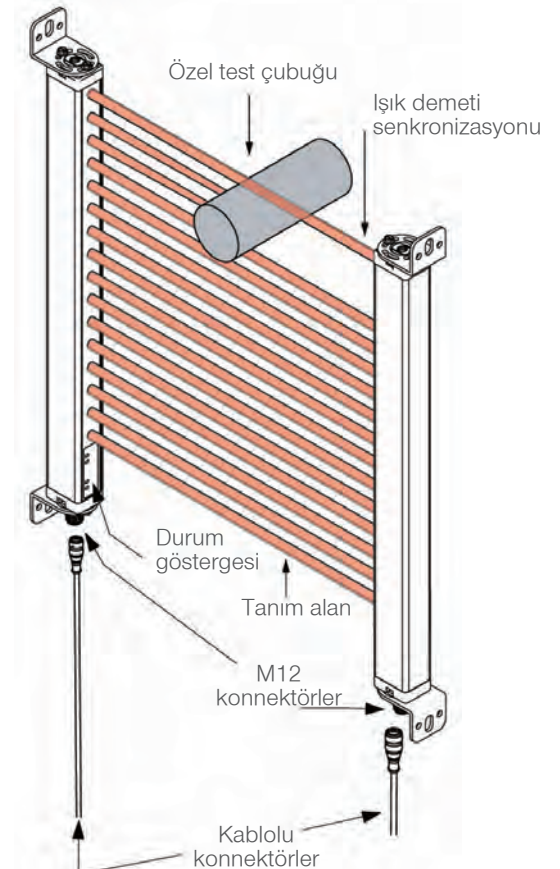
Banner EZ-Screen Tip2 Sınıfı gönderici, alıcı ve kablolu konnektörler
